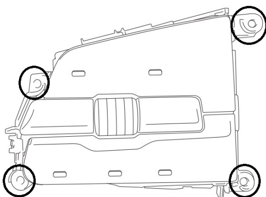
タッピングスクリュー固定部分
